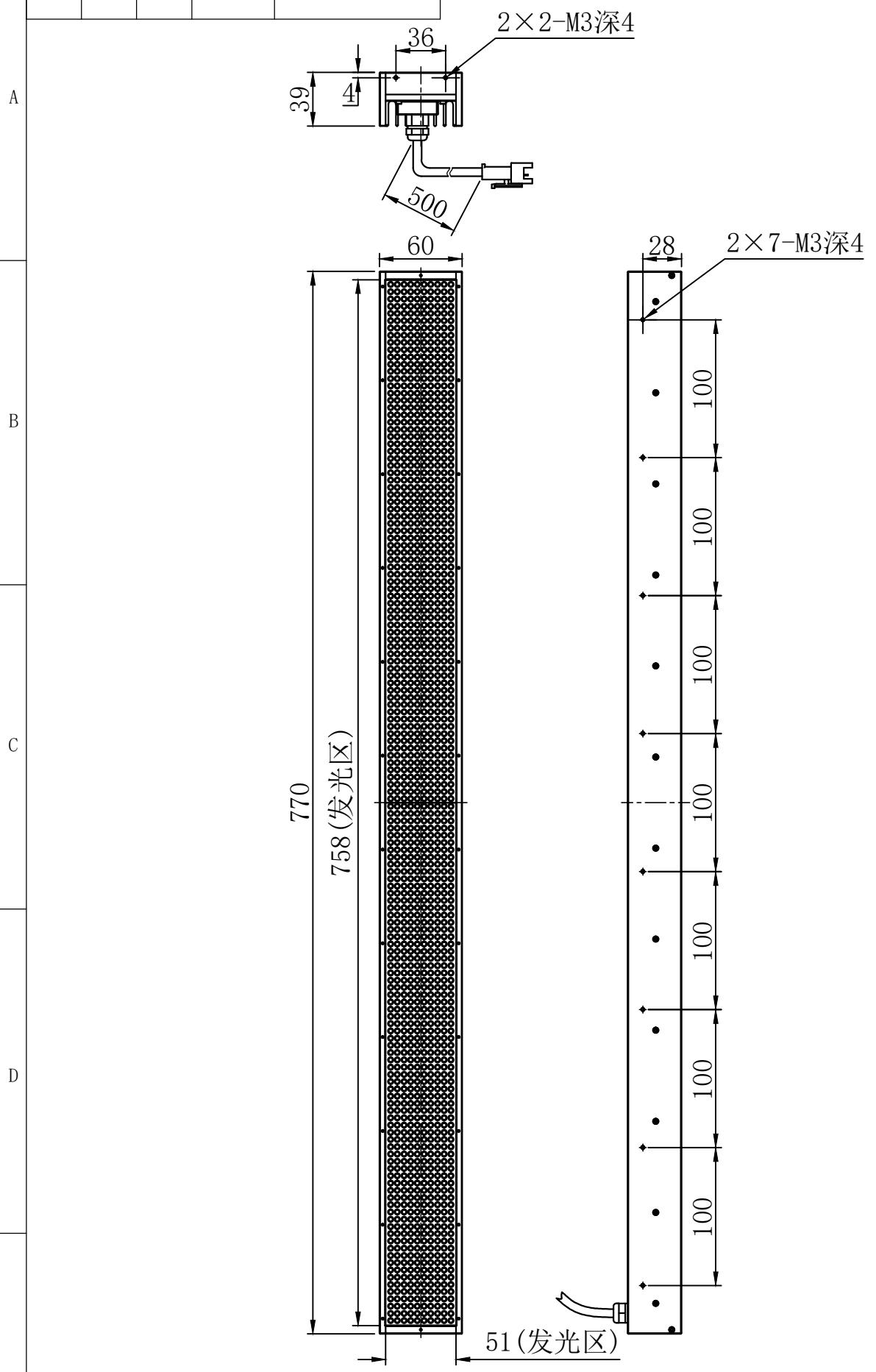
产品安装尺寸图
